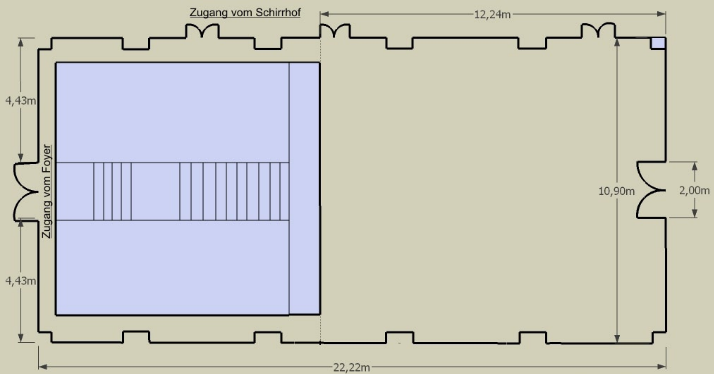
Grundriss Bühne T-Werk
